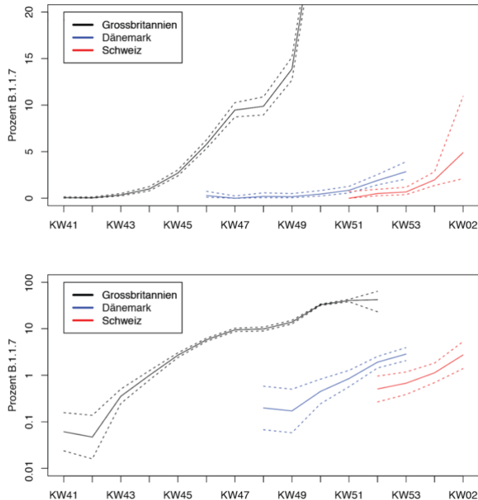
Abbildung 1: Entwicklung der Häufigkeit der B.1.1.7 Variante in Grossbritannien (schwarz), Dänemark (blau) und der Schweiz (rot). Die selben Daten sind auf einer linearen Skala (oben) und einer logarithmischen Skala (unten) dargestellt. Die untere Darstellung zeigt, dass der Anstieg in den drei Ländern ungefähr exponentiell mit einer ähnlichen Geschwindigkeit erfolgt.
